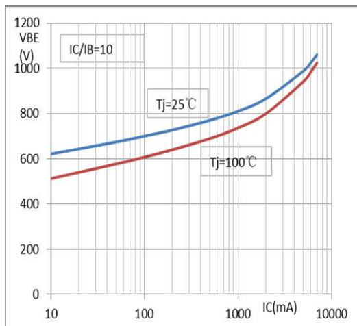
V_{BE(sat)} - I_C
